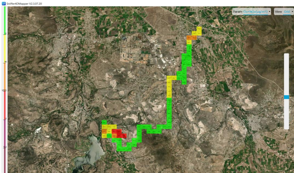
Imagen 10. Mapeo final de contaminantes en plataforma Sniffer4DMapper, Tula de Allende – PTAR Atotonilco de Tula.
