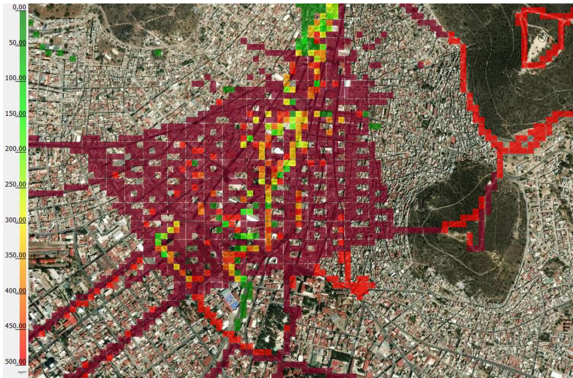
Imagen 13. Mapeo final de contaminantes en plataforma Sniffer4D-Mapper Pachuca Centro
